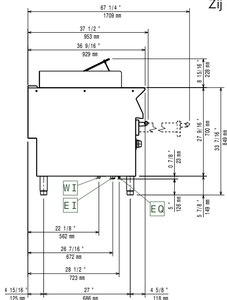
Zij aanzicht
