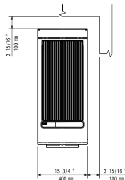
Boven aanzicht
